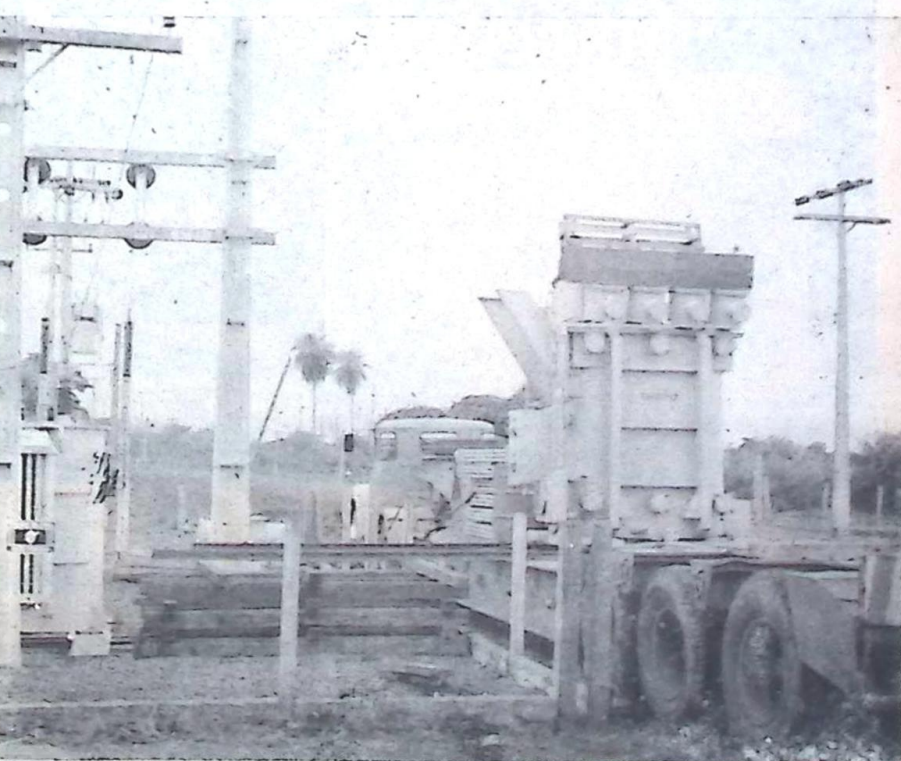
TRANSFORMADOR MAIS POTENTE PARA BELA VISTA: AGORA SÃO 3.000 KVA
