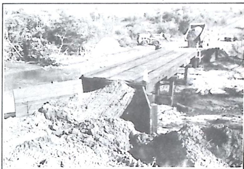
Várias pontes nas estradas vicinais do município foram recuperadas ou construídas pela atual administração, a exemplo da ponte sobre o córrego Candelão, na saída para as Caieiras
